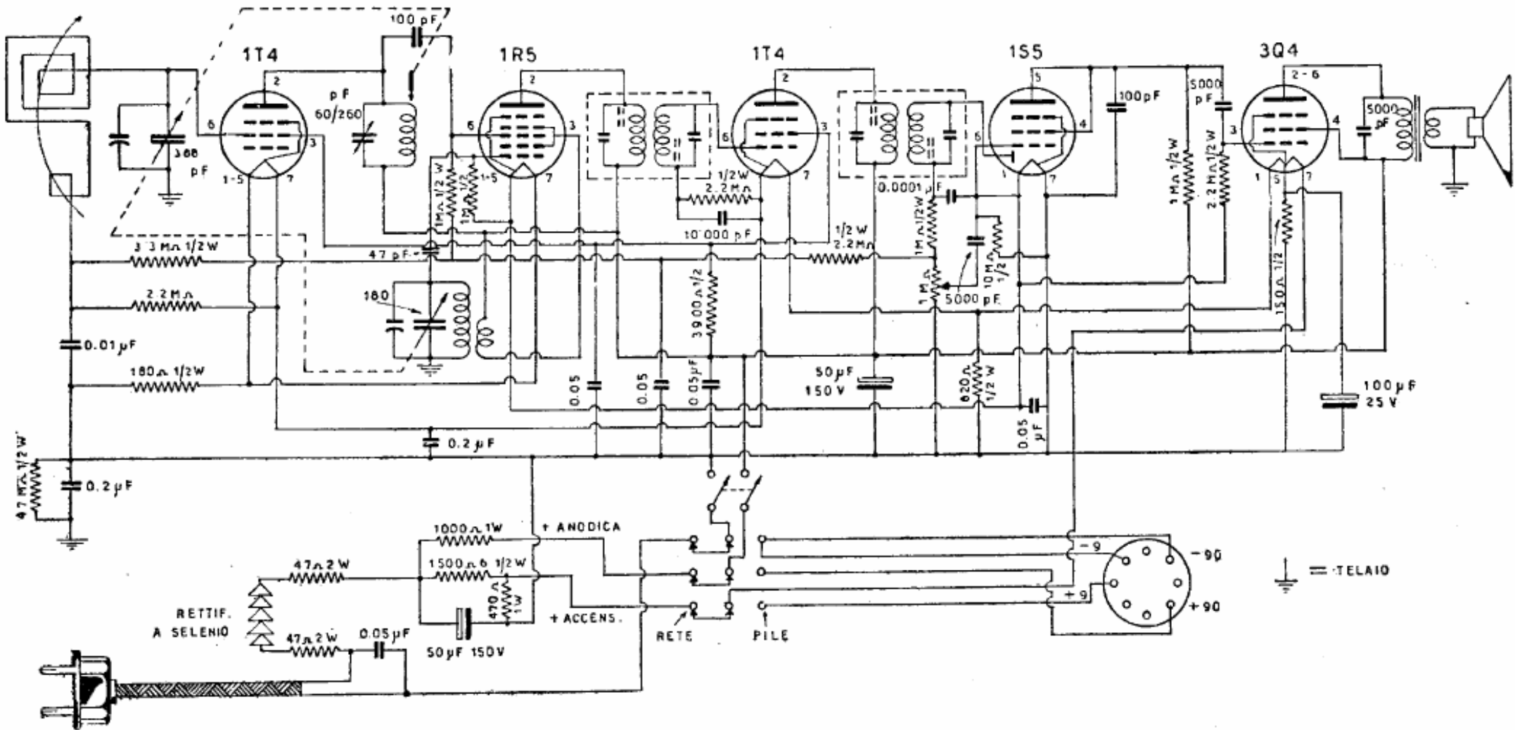
Fig. 9.12. - Schema di portatile pile-rete, con sintonia a condensatore-induttore variabili, e rettificatore a selenio
